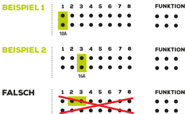
Abbildung 3. Beispiele Steckbrückenposition
