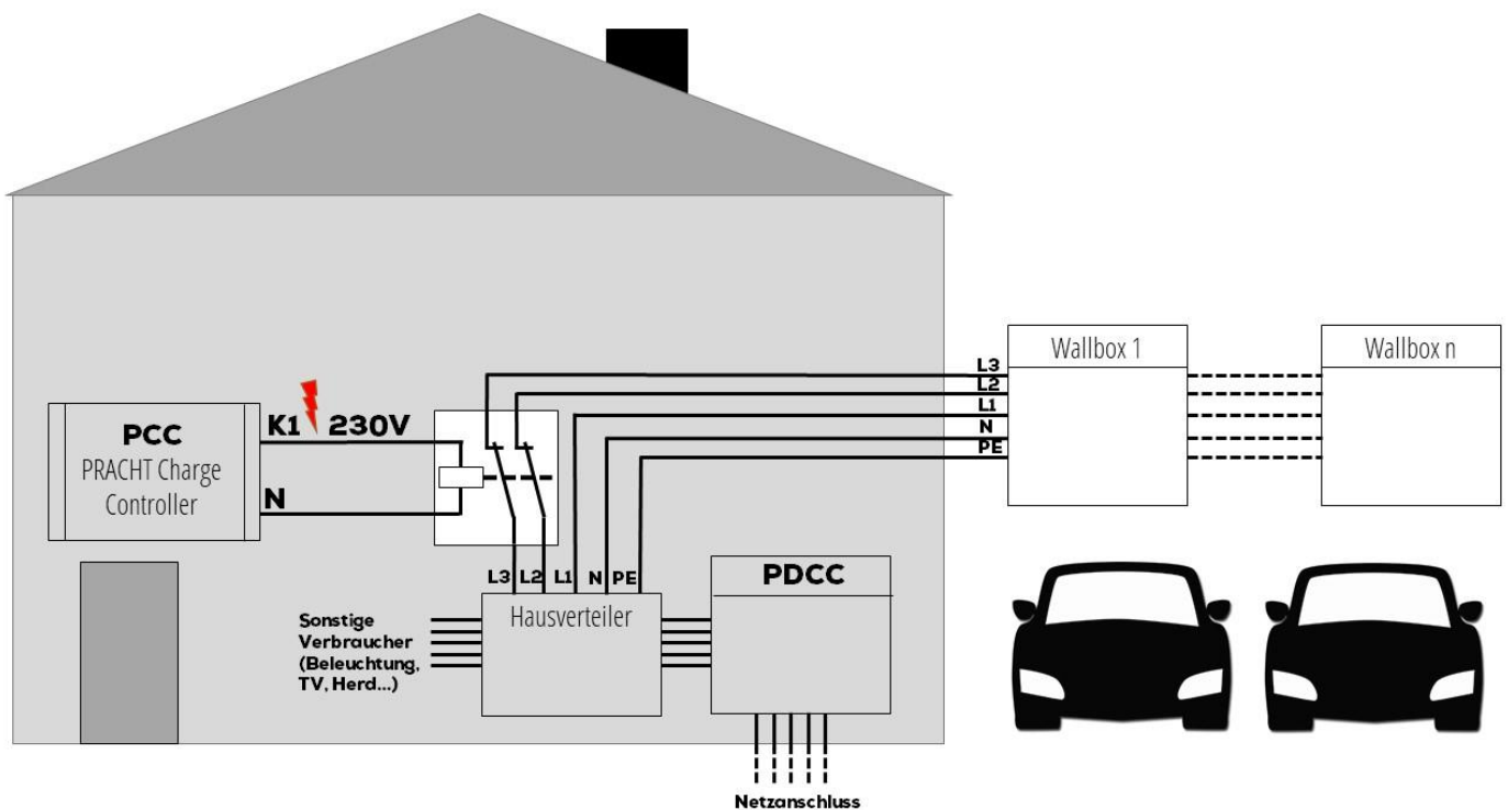
Abbildung 5 Beispiel: Phasenabwurf-Schaltung
